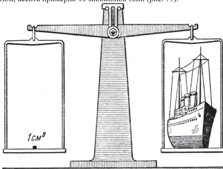
Рис. 79. Один кубический сантиметр атомных ядер мог бы уравновесить океанский пароход даже и при весьма неплотной упаковке их. Плотные же уложенные в объеме 1 \text{ см}^3 атомные ядра весили бы 10 миллионов тонн!
