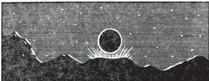
Рис. 51. «Новоземлиез» на Луне. Чёрный диск Земли окружён яркой каймой сияющей земной атмосферы.
