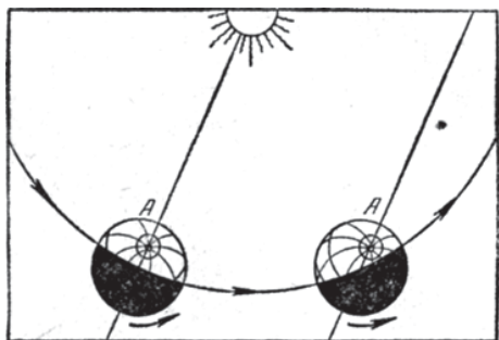
Рис. 6. Почему солнечные сутки длиннее звёздных?
