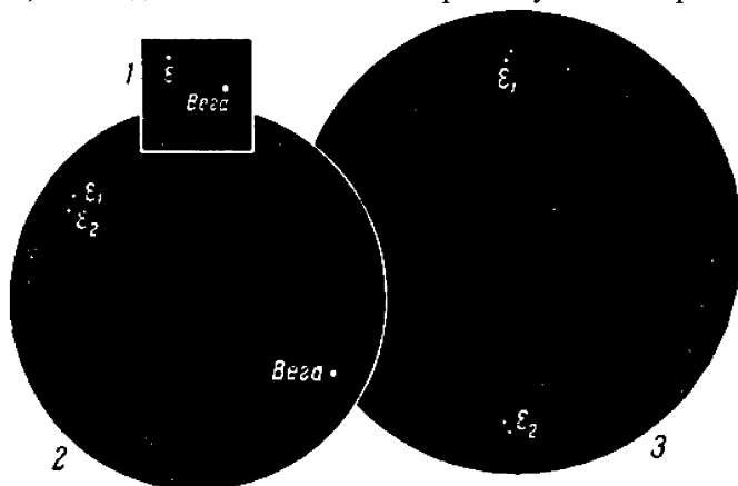
Рис. 73. Одна и та же звезда е Лиры (близ Веги), как она видна простым глазом (1), в бинокль (2) и в телескоп (3).
