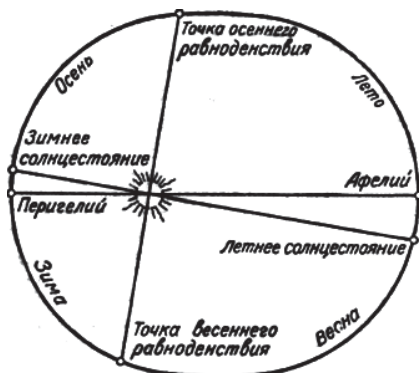
Рис. 22. Схематическое изображение пути Земли вокруг Солнца.
