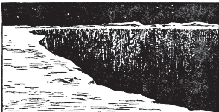
Рис. 50. Одна из лунных «трещин», наблюдаемая в непосредственной близости.
