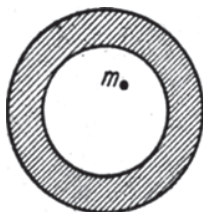
Рис. 95. Тело внутри шаровой оболочки не имеет веса.
