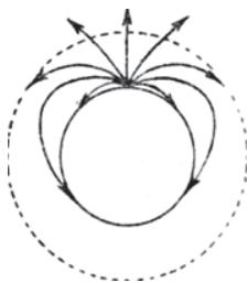
Рис. 69. Возможное скривление лучей света в атмосфере Юпитера. (О следствиях этого явления см. в тексте.)
