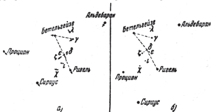
Рис. 81. В каких направлениях движутся яркие звёзды близ созвездия Ориона (а) и как эти движения изменят вид созвездия через 50 тыс. лет (б).
